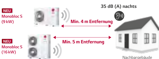
Schalldruckpegel* auf der Grundlage des Abstands zur Außeneinheit
