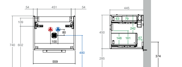
KUBE X + Unterbau 60 cm 2 Auszüge, soft-close Art. Nr. JR999/7331 WUKXP60CX*
