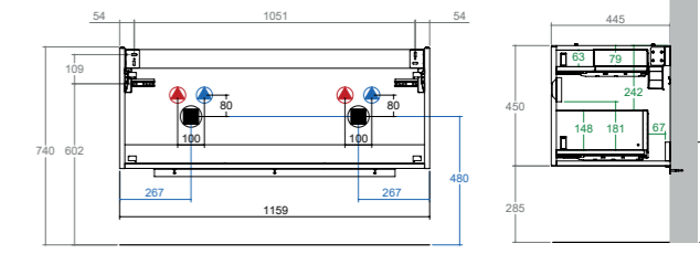
KUBE X + Unterbau 120 cm 2 Auszüge, soft-close Art. Nr. JR999/7331 WUKXP12D2X*
