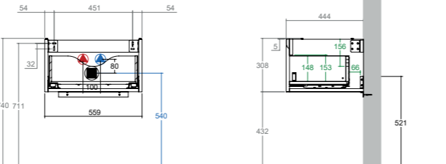
KUBE X + Unterbau 60 cm 1 Auszug, soft-close Art. Nr. JR999/7331 WUKXP601CX*
