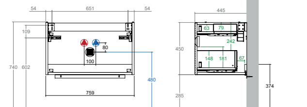
KUBE X + Unterbau 80 cm 1 Auszug, soft-close Art. Nr. JR999/7331 WUKXP801CX*
