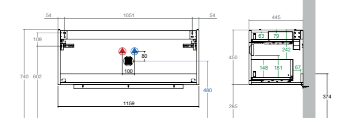
KUBE X + Unterbau 120 cm 2 Auszüge, soft-close Art. Nr. JR999/7331 WUKXP120CX*
