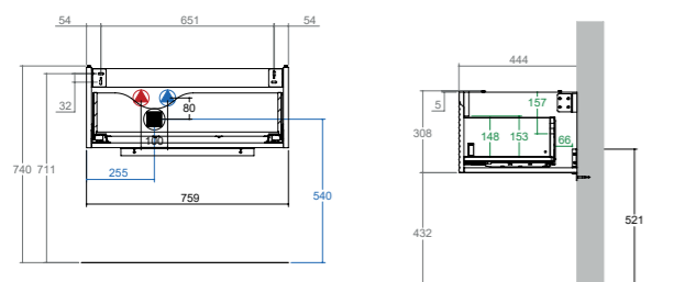
KUBE X + Unterbau 80 cm 1 Auszug, soft-close, Becken links Art. Nr. JR999/7331 WUKXP801SX*
