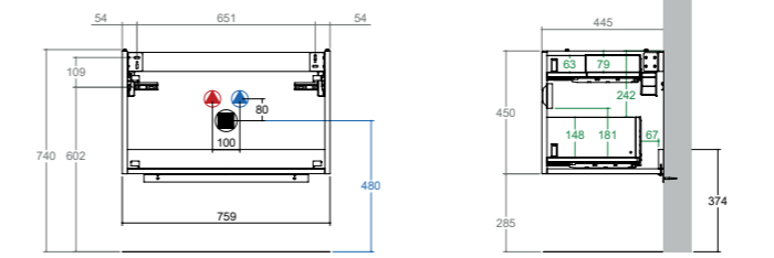
KUBE X + Unterbau 80 cm 2 Auszüge, soft-close Art. Nr. JR999/7331 WUKXP80CX*
