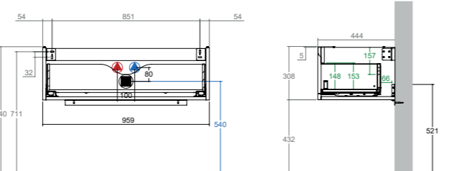
KUBE X + Unterbau 100 cm 1 Auszug, soft-close Art. Nr. JR999/7331 WUKXP1001CX*
