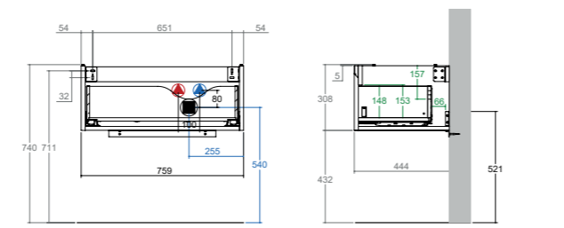
KUBE X + Unterbau 80 cm 1 Auszug, soft-close, Becken rechts Art. Nr. JR999/7331 WUKXP801DX*
