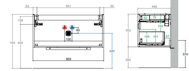
KUBE X + Unterbau 100 cm 2 Auszüge, soft-close Art. Nr. JR999/7331 WUKXP100CX*
