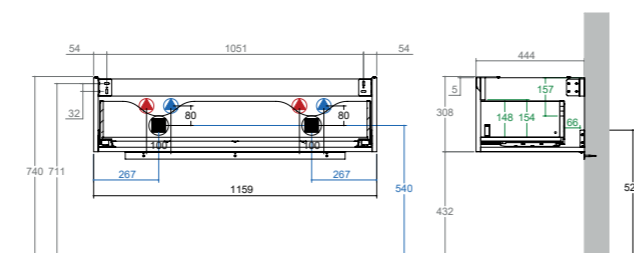
KUBE X + Unterbau 120 cm 1 Auszug, soft-close Art. Nr. WUKXP12D11X*
