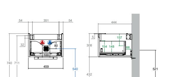
KUBE X + Unterbau 50 cm 1 Auszug, soft-close Art. Nr. JR999/7331 WUKXP501CX*
