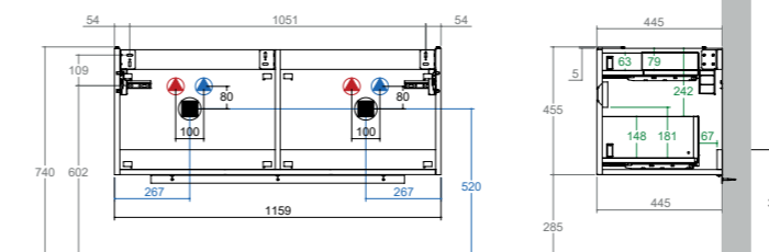
KUBE X + Unterbau 120 cm 4 Auszüge, soft-close Art. Nr. JR999/7331 WUKXP12D4X*
