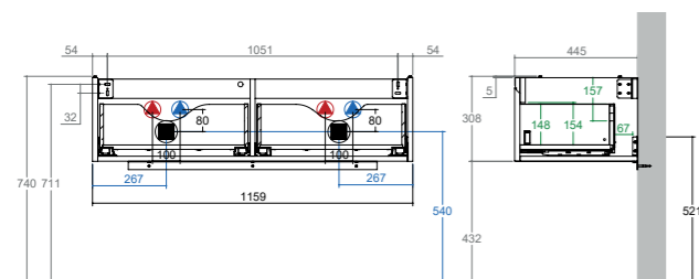
KUBE X + Unterbau 120 cm 2 Auszüge, soft-close Art. Nr. JR999/7331 WUKPX12D12X*
