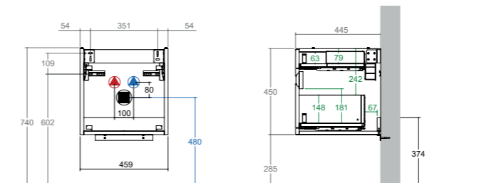
KUBE X + Unterbau 50 cm 2 Auszüge, soft-close Art. Nr. JR999/7331 WUKXP50CX*
