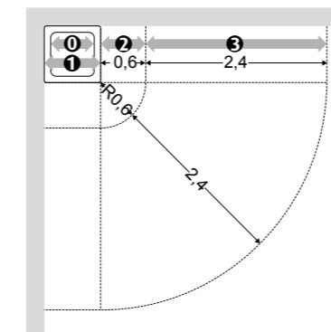
Bereichseinteilung bei Räumen mit Duschwanne
