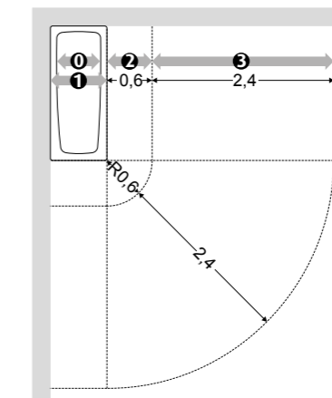
Bereichseinteilung bei Räumen mit Badewanne
